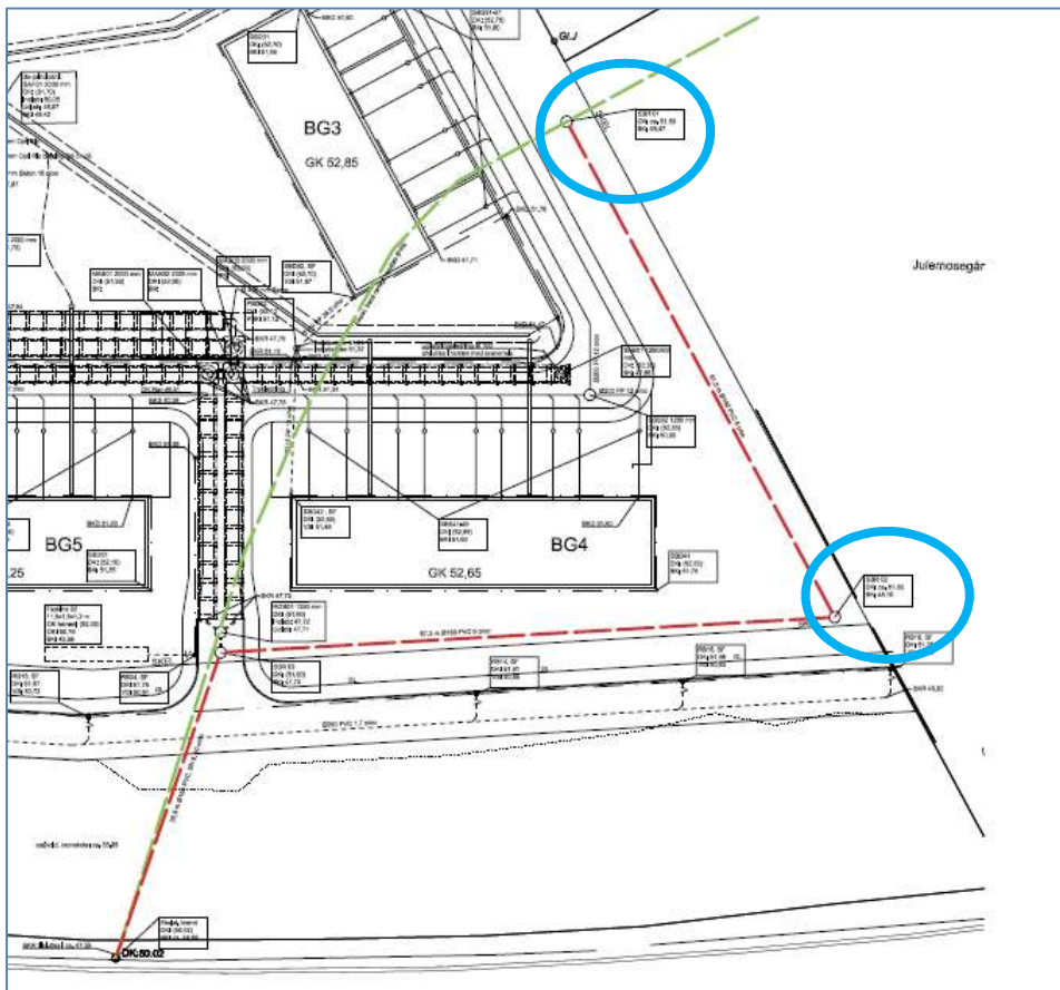
Figur 2. Udsnit af Tegning nr.: JUL_K10_H1_EST_01 suppleret med blå farvemarkering af vandløbsbrønde SBR_01 og SBR_02. Tegning er udarbejdet i forbindelse med byggeriet af Julemoesvænge 1-73, beliggende vest for Julemoesgård. Vandløbsbrønd SBR_01 og SBR_02 er beliggende på den røde stiplede linje, der illustrerer placeringen af det privat rørlagt vandløb, nord for Slangerupvej. Den grønne stiplede linje markerer den oprindelige placering af vandløbet før byggeselskabet af Julemoesvænge 1-73. Nærmere detaljer om brønd SBR_01 og SBR_02 ses af bilag 1.
